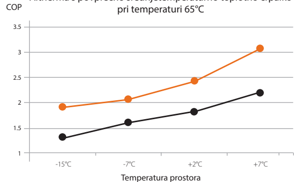
Primerjava visokotemperaturne toplotne črpalke Daikin Altherma s povprečno srednjetermperaturno toplotno črpalko pri temperaturi 65°C
